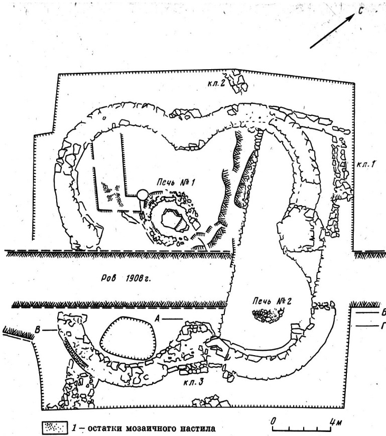
Рис. VII. 1. План четырехапсидного храма по В.А.Кутайсову
