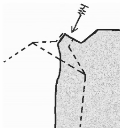
Рис. 43. Подготовка точки для приложения импульса силы в зоне сопряжения ударной площадки и фронта скалывания
