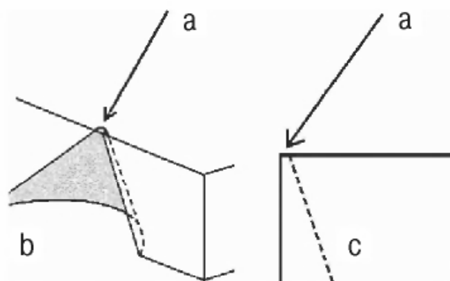
Рис. 62. Направление вектора расщепляющей камень силы (a) и реальная конфигурация конусовидной трещины в изометрии (b) и в плане (c)
