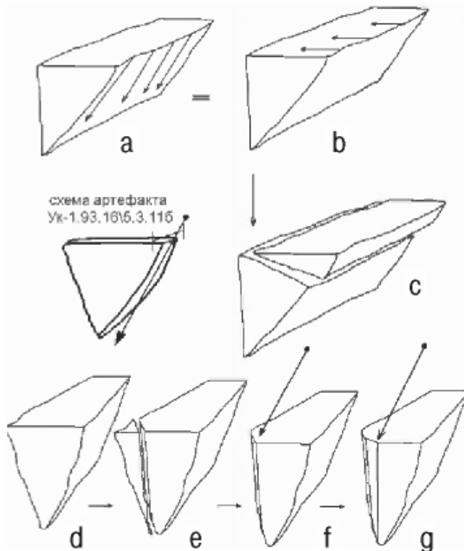
Рис. 92. Схема основных снятий (а), снятий оживления (b), удаления объёма на ударной площадке (с) и начало торцового расщепления (d-f) плиточных форм сырья на памятнике Усть-Каракол I
