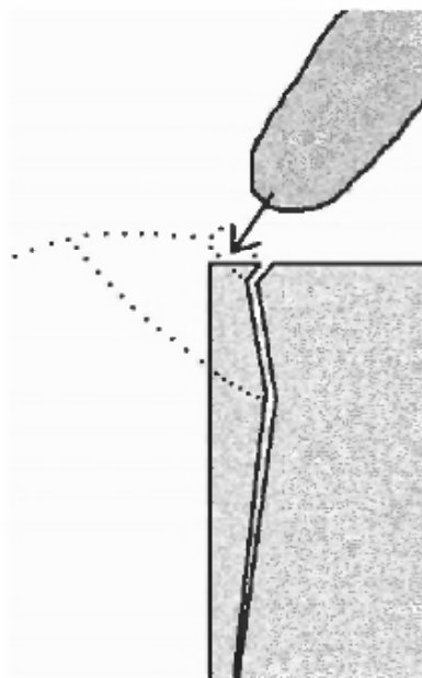
Рис. 31. Последствия приложения импульса силы под углом к ударной площадке
