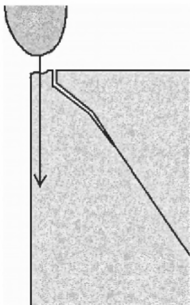
Рис. 30. Последствия приложения импульса силы перпендикулярно ударной площадке
