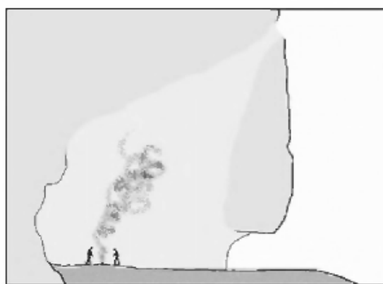
Рис. 3. Денисова пещера
