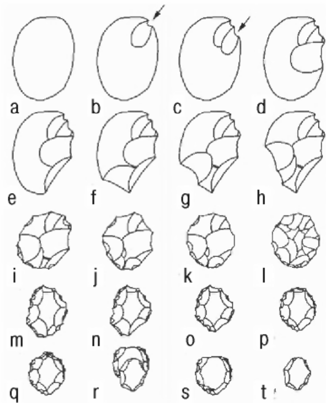
Рис. 103. Один из вариантов схемы расщепления леваллуа (подготовка пренуклеуса (a–q); основное снятие (r); нуклеус (s) и «отщеп леваллуа» (t)
