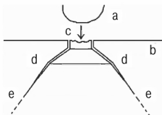
Рис. 24. Схема формирования конусной трещины: отбойник (а), расщепляемый камень (б), «таблетка» (с), развитие (d) и угасание (e) трещины
