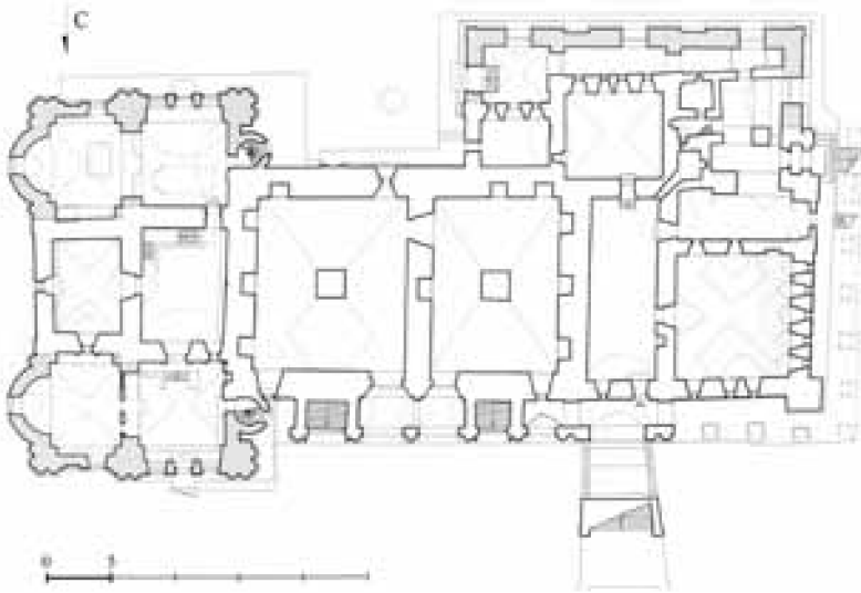
Новая трапезная. План 1-го этажа. Штриховкой показаны объёмы, пристроенные в XIX веке. Проект реставрации с восстановлением части галереи. Чертёж А.О. Дмитриевой
