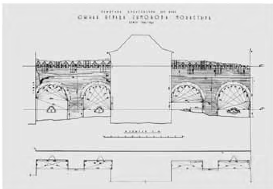
Южное прясло стены. Обмер. 1950-е гг.
