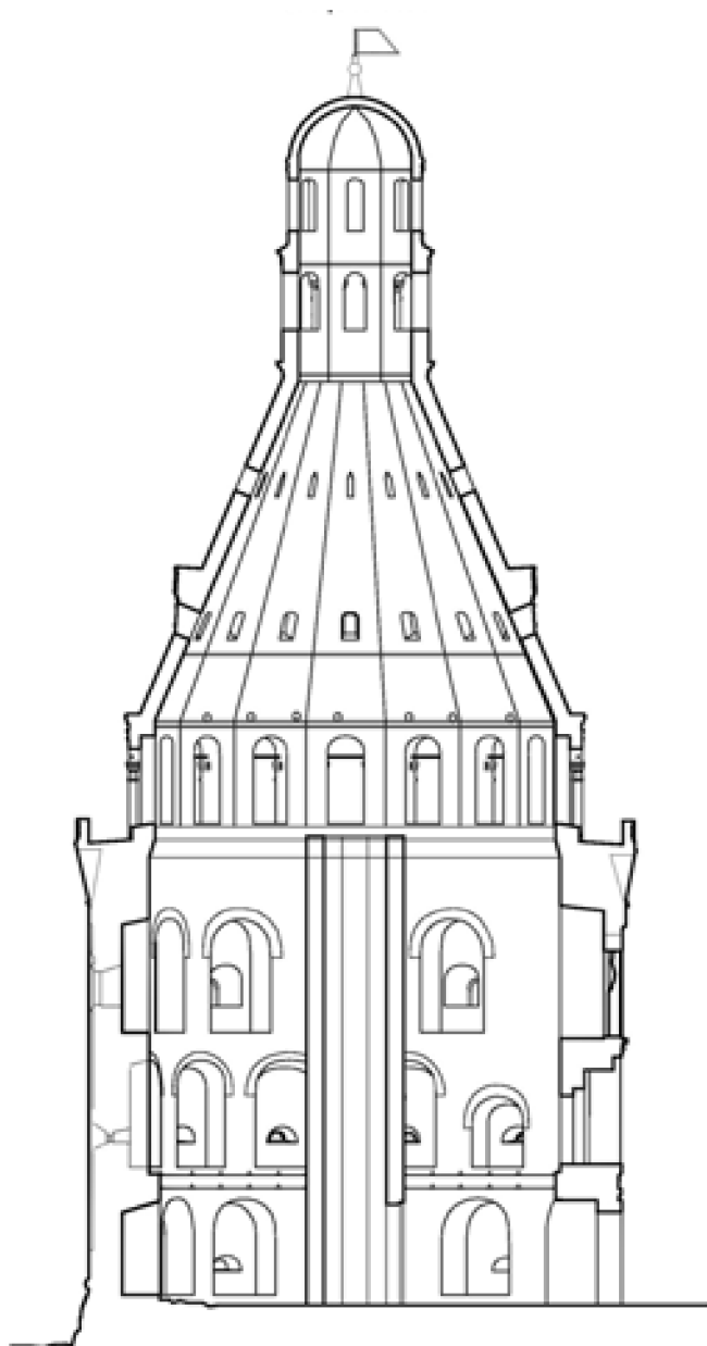
Башня Дуло. Разрез 1-1. Чертёж Е.А. Александровой
