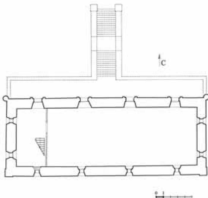
Сушило. План 2-го этажа с графической реконструкцией галереи. Штриховкой показана современная кладка. Чертёж А.И. Винокуровой
