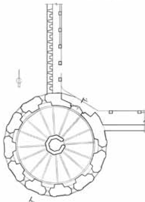
Башня Дуло. План второго яруса. Чертёж Е.А. Александровой
