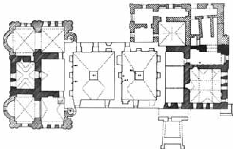
Новая трапезная. План стен в подвале. Обмеры арх. Эрн и Харламовой. ГНИМА, Г-2423
