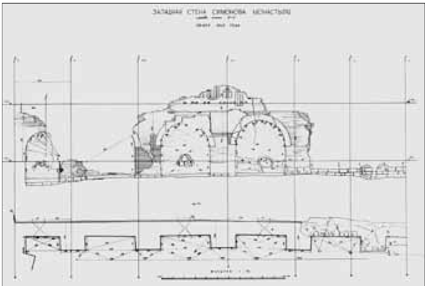
Фрагмент западного прясла стены. Обмер. 1950-е гг.
