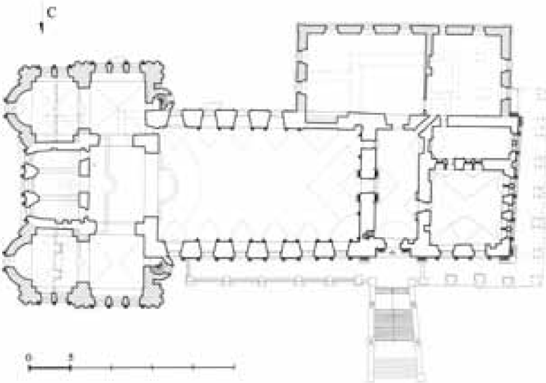
Новая трапезная. План 2-го этажа. Штриховкой показаны объёмы, пристроенные в XIX веке. Проект реставрации с восстановлением части галереи. Чертёж А.О. Дмитриевой
