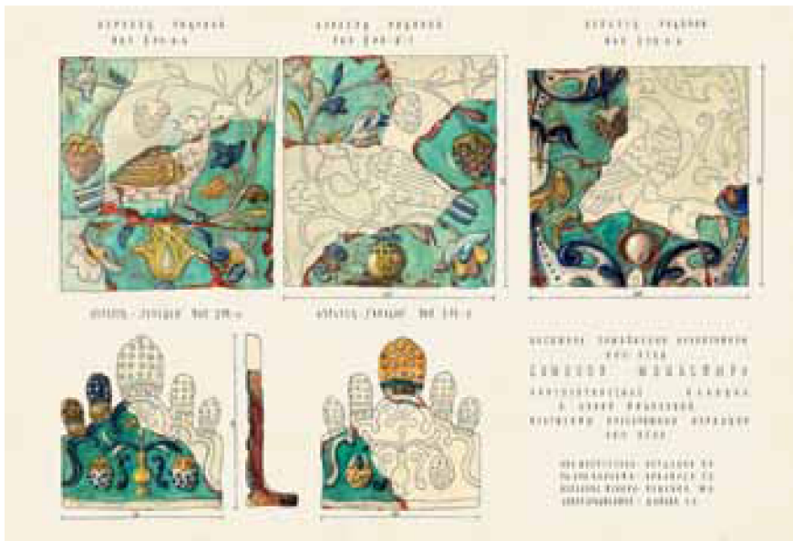
31. Новая трапезная. Изразцы печного набора. Чертёж М.О. Пушкиной
