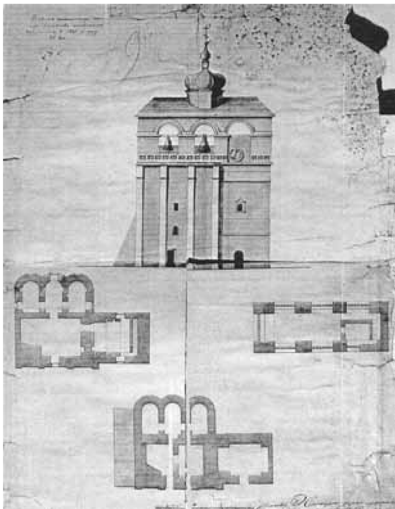
Звонница. Фасад и планы. Чертёж нач. XIX в. Арх. Корольков. ГНИМА, РІ-1085; V-41422, V-39116, XIII-1528
