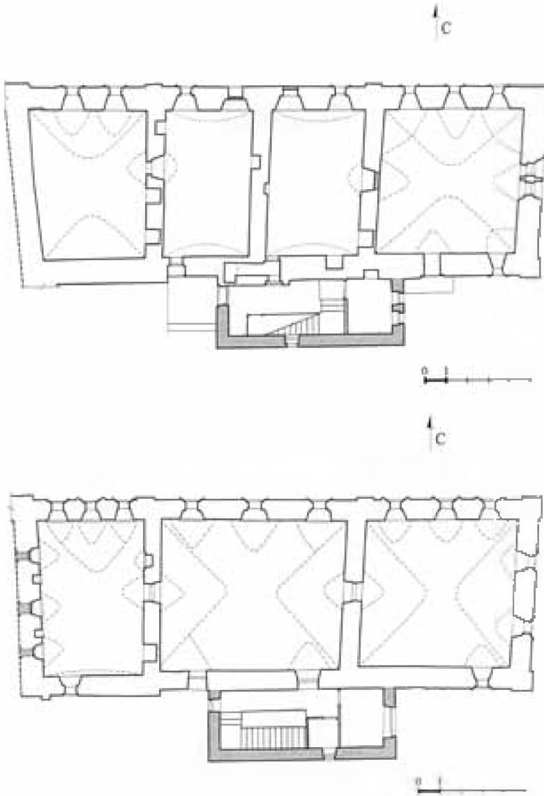
Казначейский корпус. План 1-го этажа. Штриховкой показана современная кладка. Чертёж Е.Ю. Солоухиной
