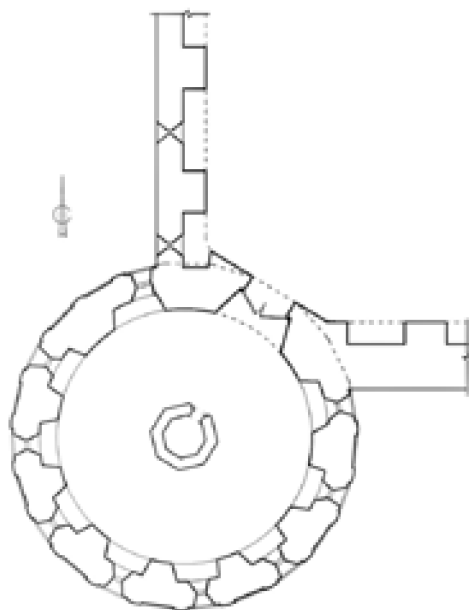
Башня Дуло. План первого яруса. Чертёж Е.А. Александровой
