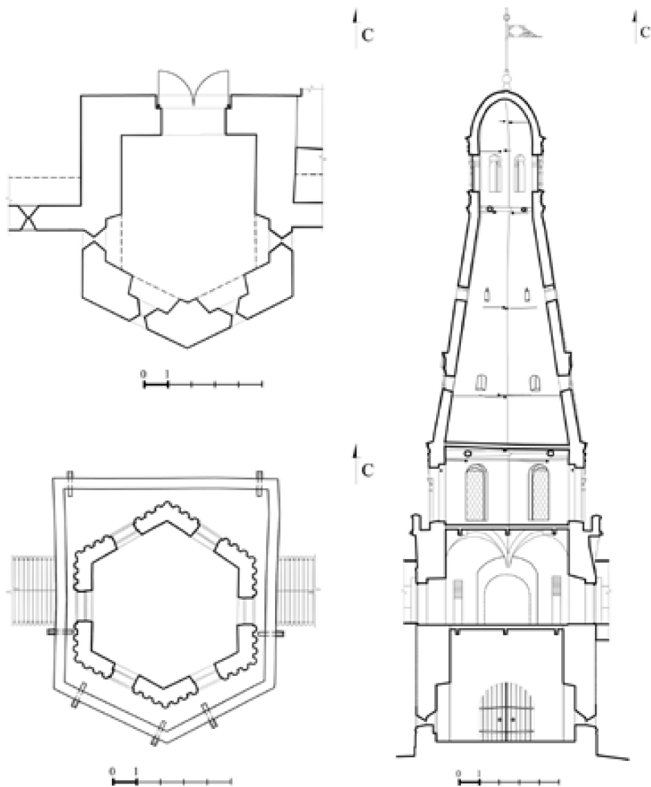
Кузнечная башня. Разрез (существующие лестницы условно не показаны). Видны конструкции, встроенные при возведении шатра. Чертёж Н.П. Александровой
