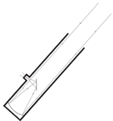
Рефлектор Ньютона
