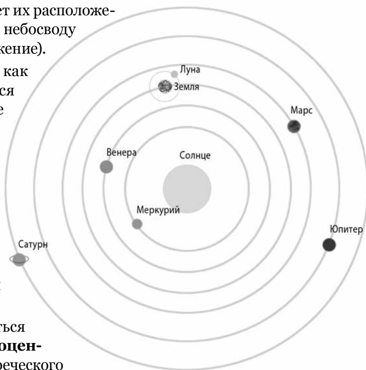
Гелиоцентрическая модель
