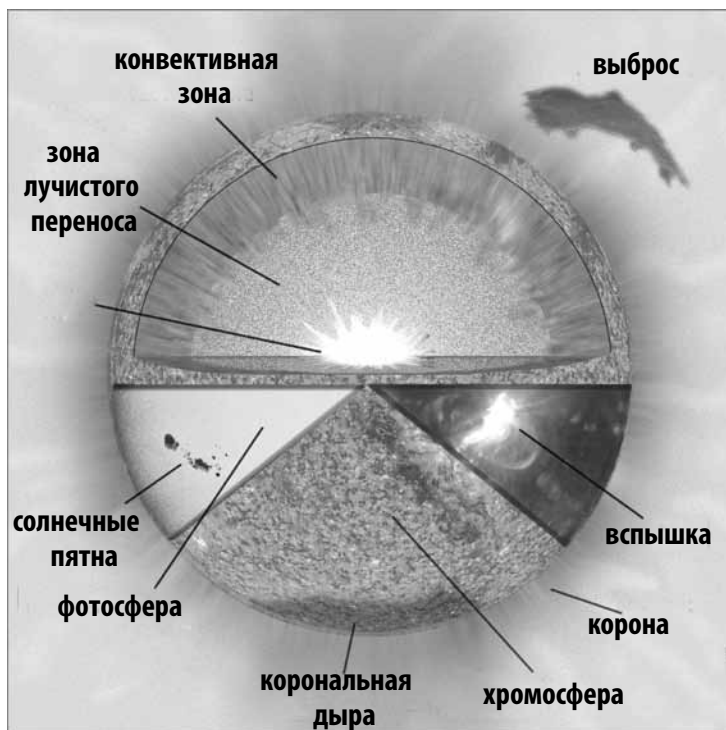
Строение Солнца
