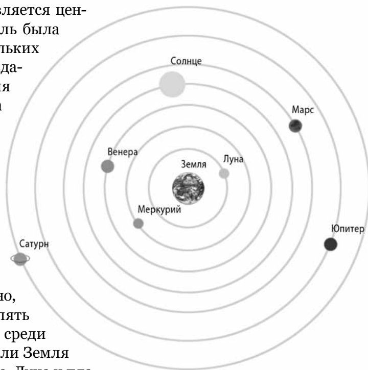
Геоцентрическая модель
