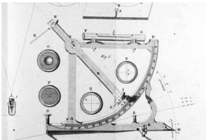
Квадрант
