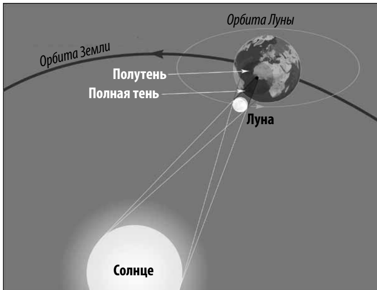
Полное солнечное затмение
